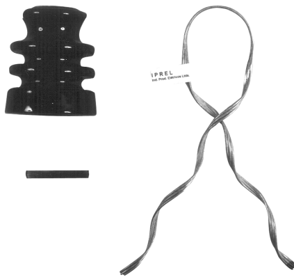
Pesçoço do Isolador 75mm/Cuello del aislador 75mm/Insulator neck 2-7/8"
